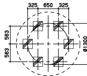
基礎伏図 S=1/50
