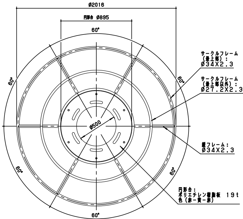
平面図 S=1/20
