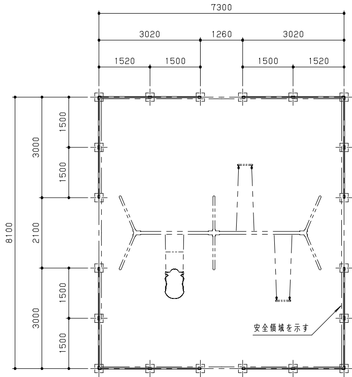
平面図 S = 1/80
