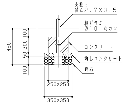
基礎断面詳細図 S = 1/20
