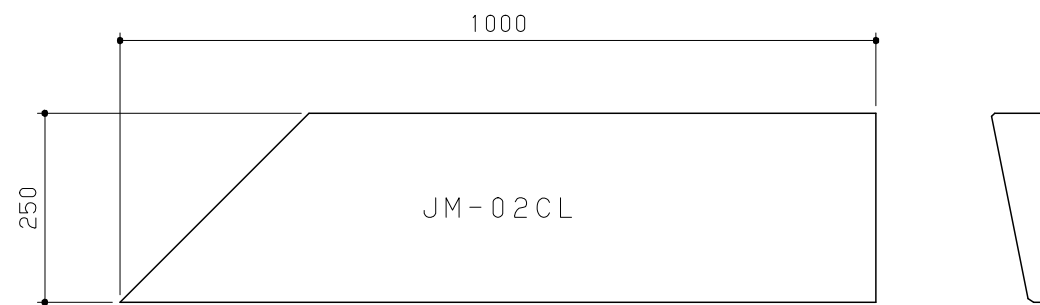
平面図 S = 1 / 10
