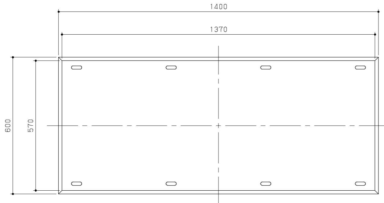
平面図 S = 1 / 10
