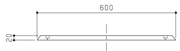
側面図 S = 1 / 10
