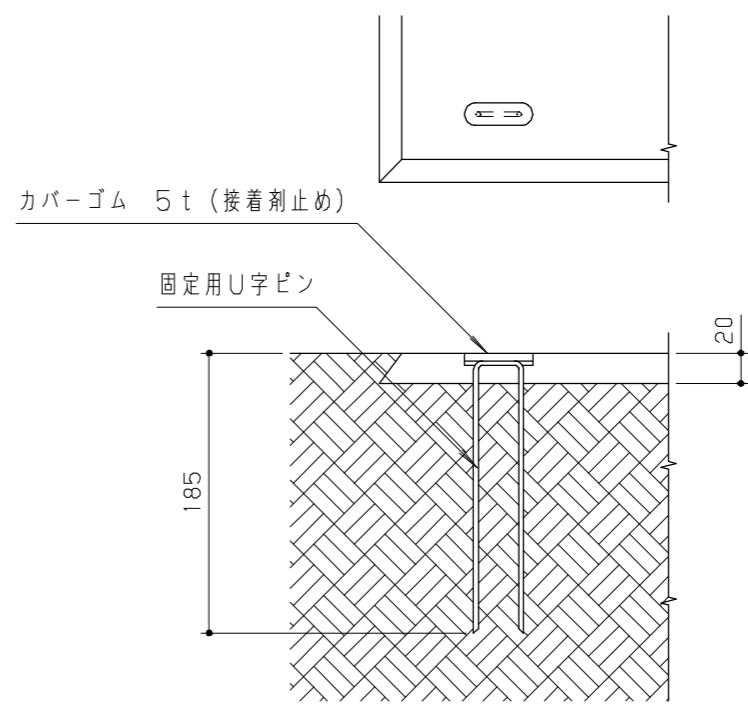
設置標準図 S = 1 / 5
