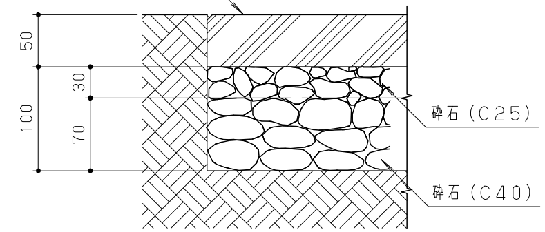
設置参考図 S = 1 / 5
