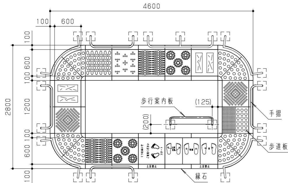
平面図 S = 1 / 50
