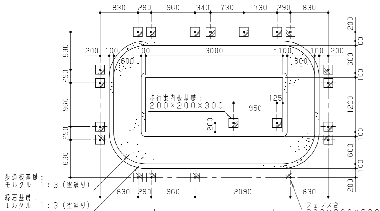
基礎伏図 S = 1 / 50
