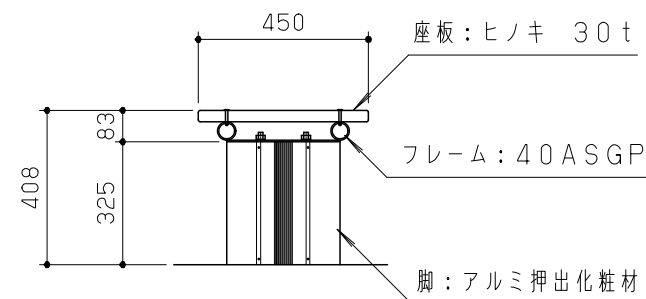
断面図 S=1/20
