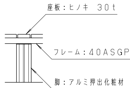
立面図 S=1/20
