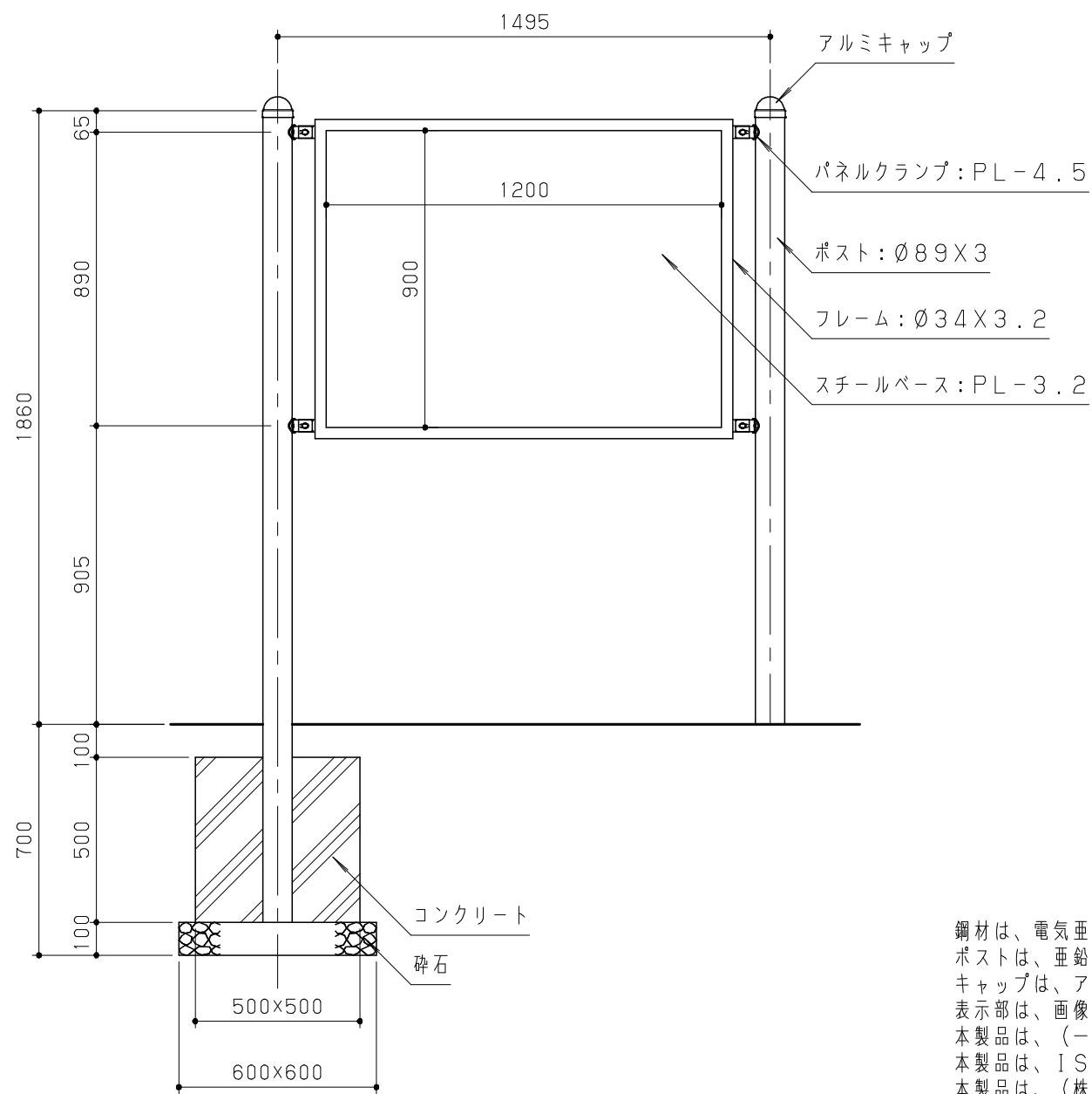
立面図 S = 1 / 20
