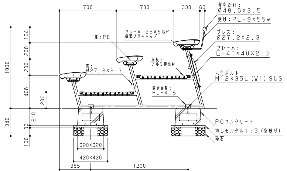
断面図 S=1/20
