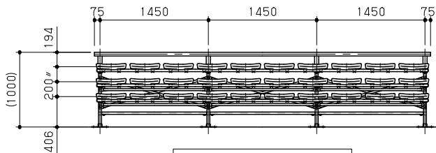
立面図 S=1/50
