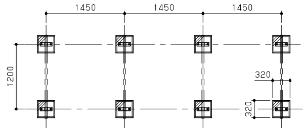
基礎伏図 S=1/50
