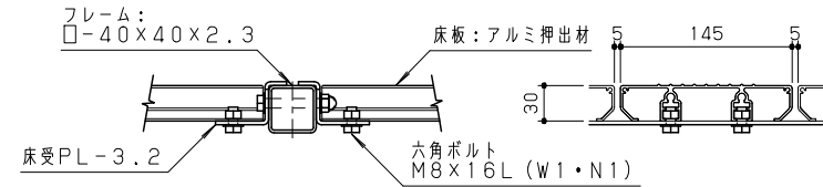
床板取付標準図 S=1/5
