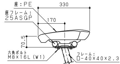
ベンチ標準断面図 S=1/10
