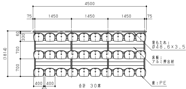
平面図 S=1/50
