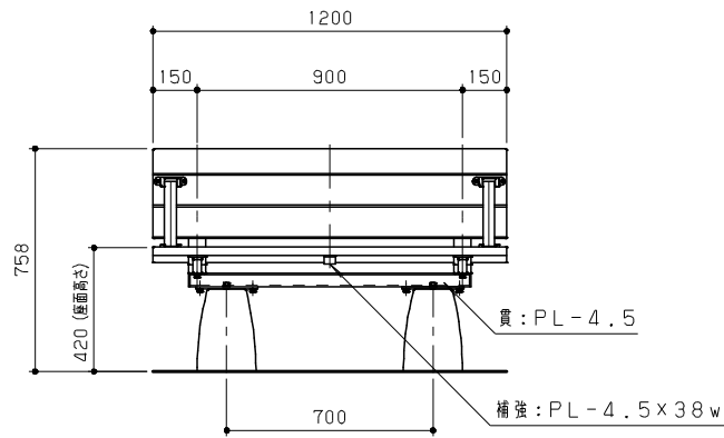
立面図 S = 1/20
