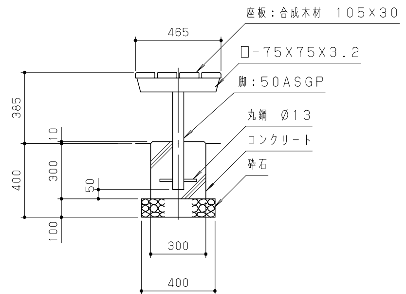
側面図 S = 1/20
