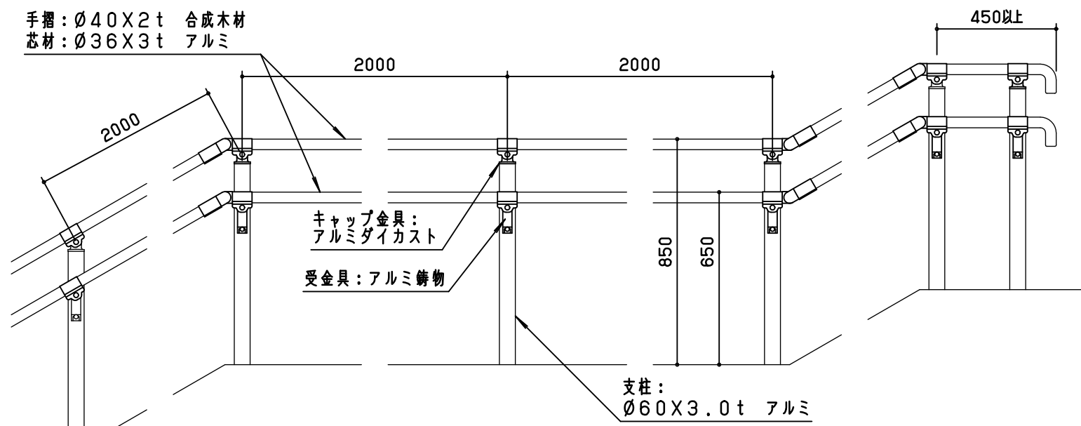
標準立面図 S = 1 / 20
