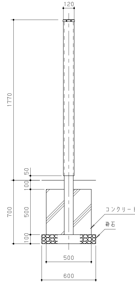
側面図 S = 1/20
