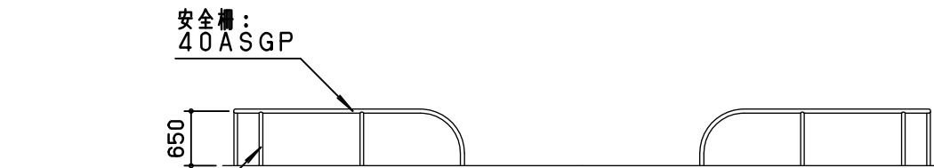
側面図 S=1/80
