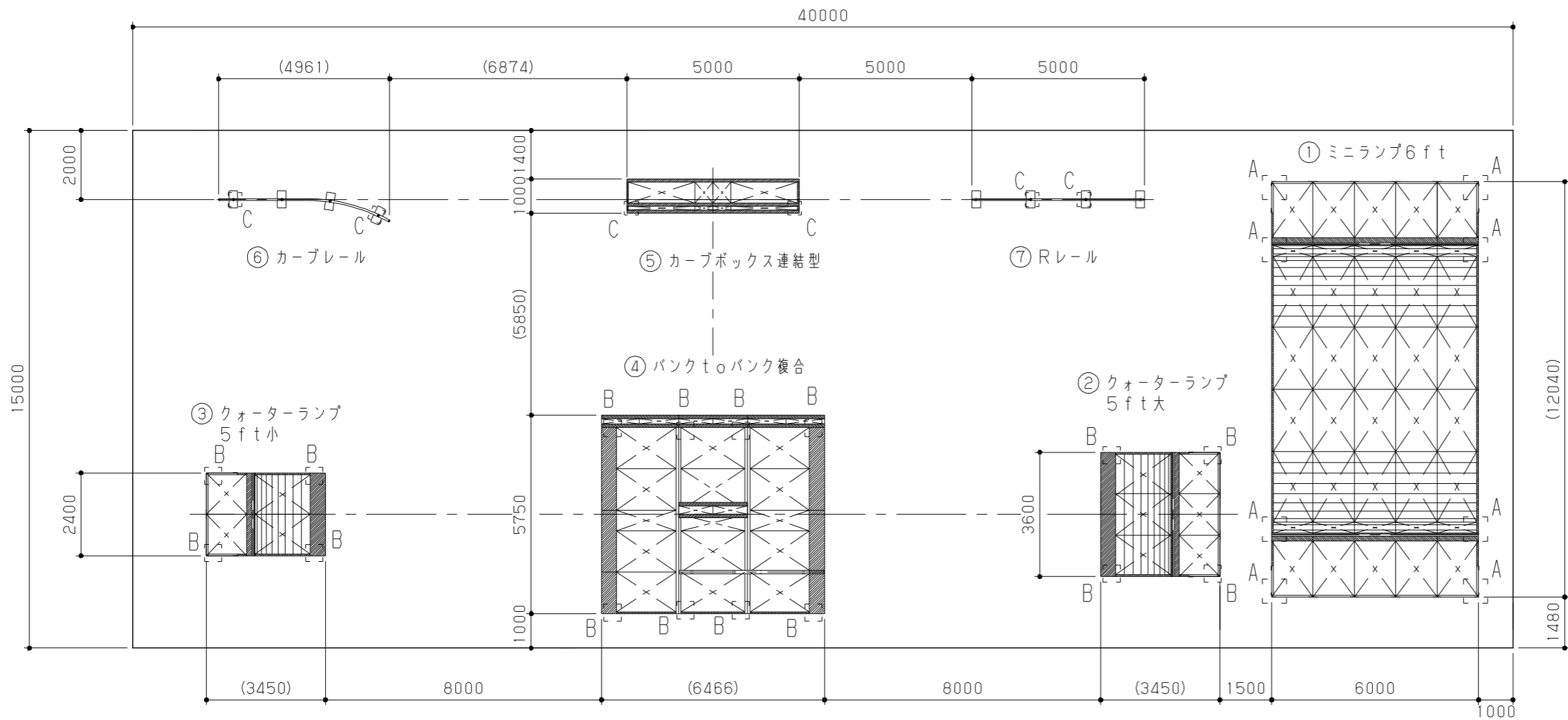
平面配置図 S=1/150
