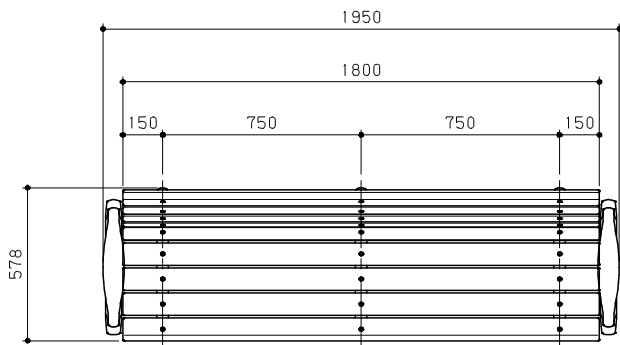
平面図 S = 1/20
