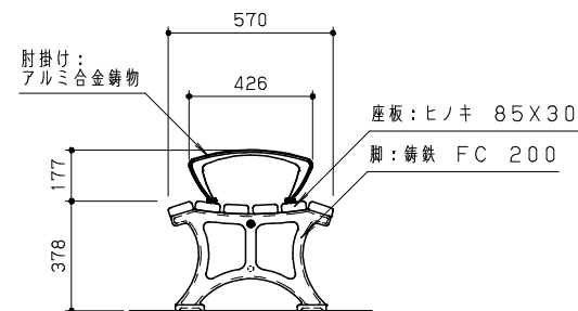
側面図 S = 1 / 20
