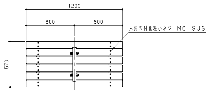
平面図 S = 1 / 20
