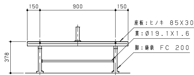
正面図 S = 1 / 20
