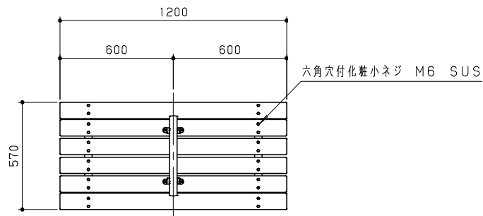
平面図 S=1/20
