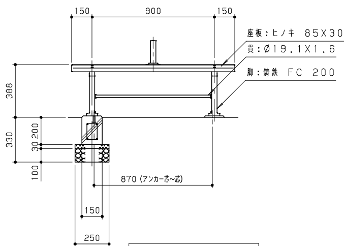
正面図 S=1/20
