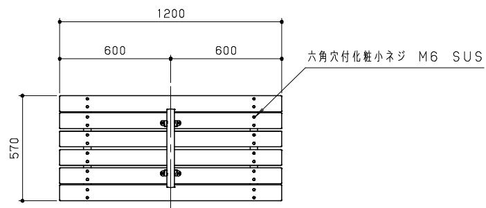
平面図 S = 1 / 20
