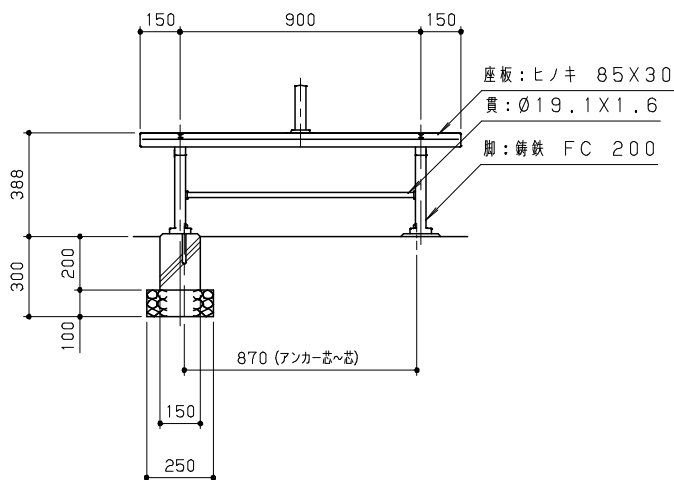
正面図 S = 1 / 20
