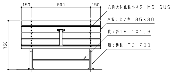
正面図 S=1/20
