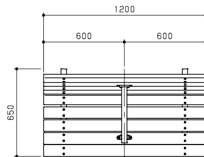
平面図 S=1/20
