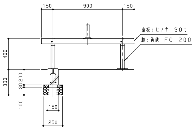
正面図 S=1/20
