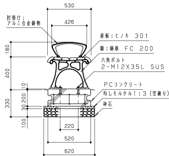
側面図 S=1/20
