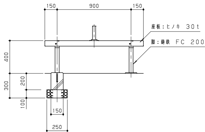
正面図 S=1/20
