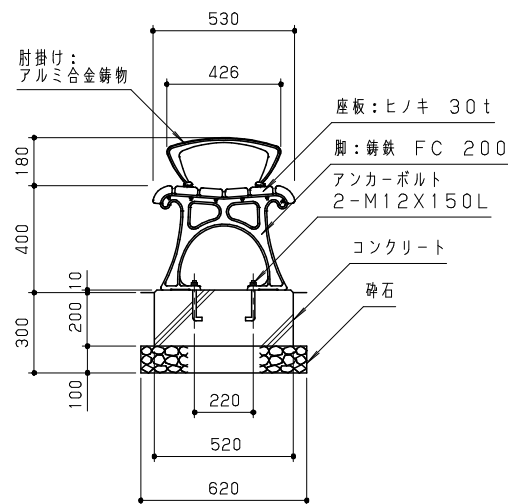
側面図 S=1/20
