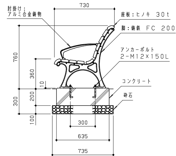
側面図 S = 1 / 20
