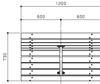
平面図 S = 1 / 20
