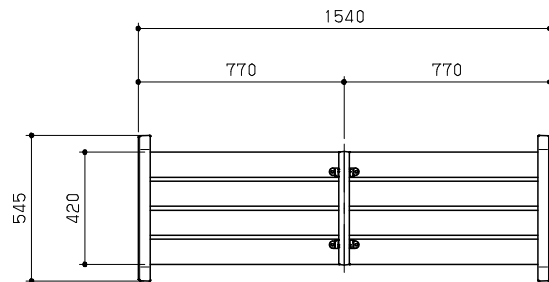
平面図 S = 1 / 20
