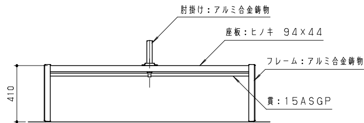
立面図 S = 1 / 20
