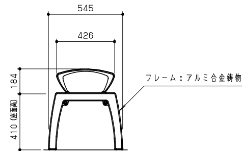
側面図 S = 1 / 20
