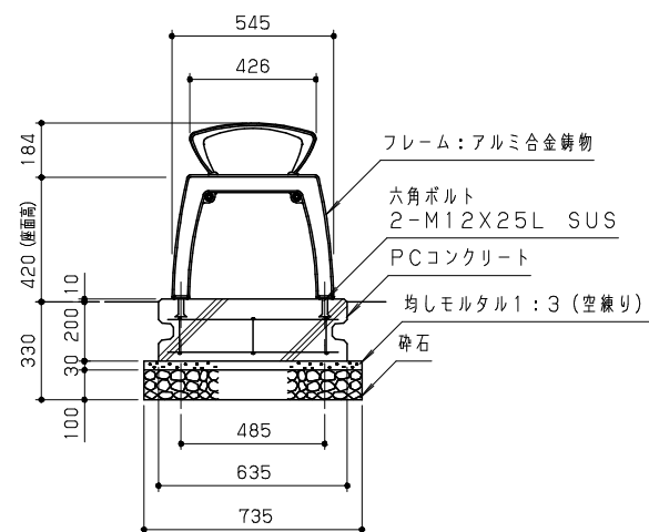
側面図 S=1/20
