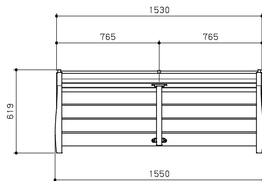
平面図 S=1/20
