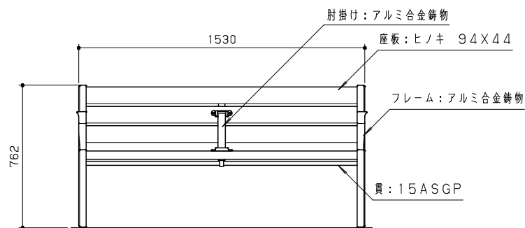
立面図 S=1/20
