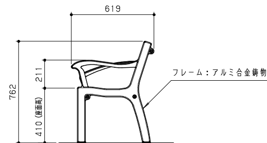
側面図 S=1/20
