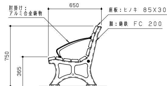
側面図 S = 1 / 20
