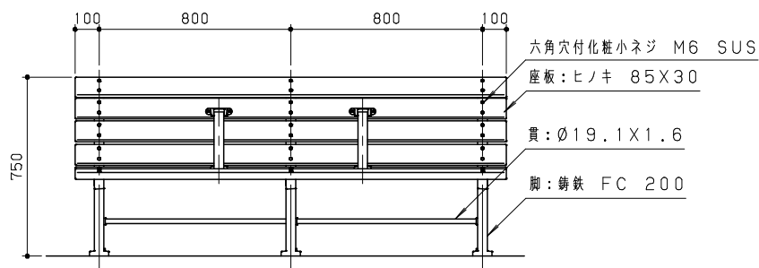
正面図 S = 1 / 20
