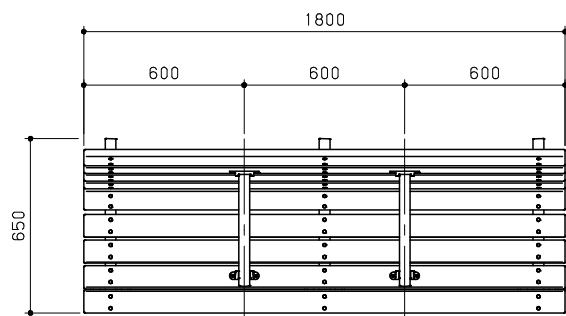
平面図 S = 1 / 20
