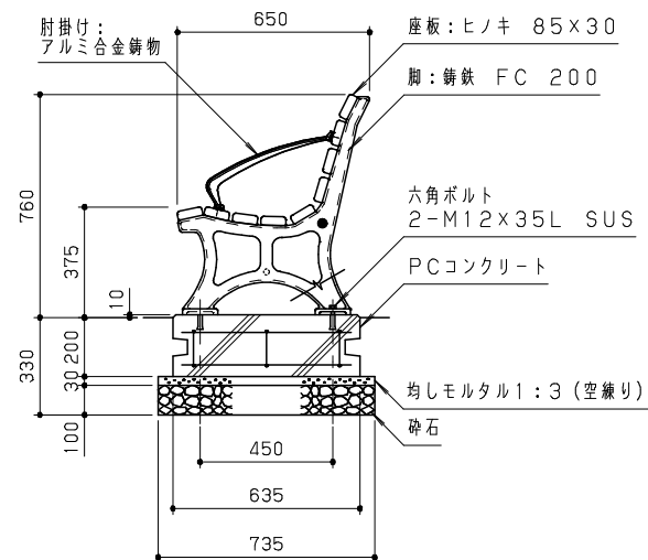
側面図 S = 1 / 20
