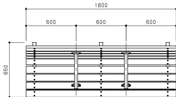
平面図 S = 1 / 20
