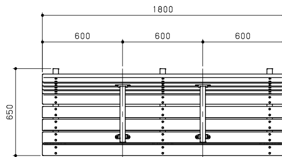
平面図 S = 1 / 20
