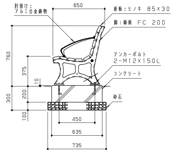
側面図 S = 1/20
