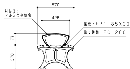
側面図 S = 1 / 20
