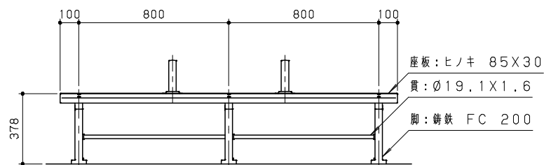
正面図 S = 1 / 20
