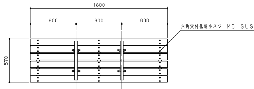
平面図 S = 1 / 20
