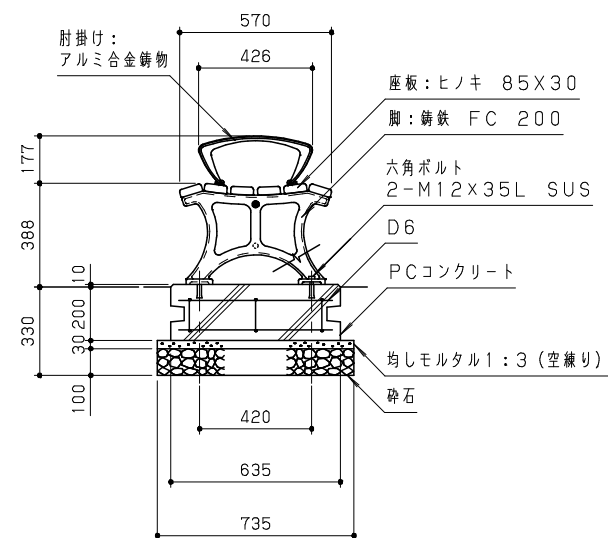
側面図 S = 1 / 20
