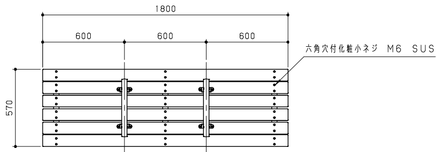
平面図 S=1/20
