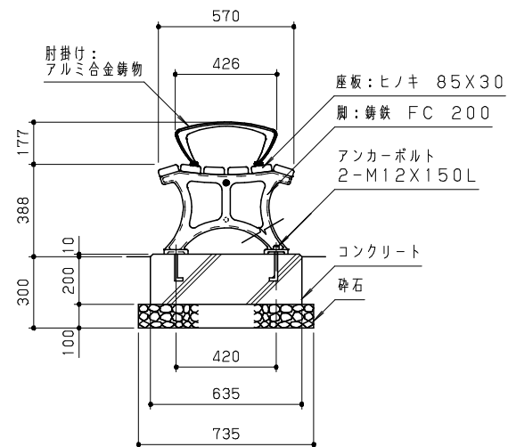
側面図 S=1/20
