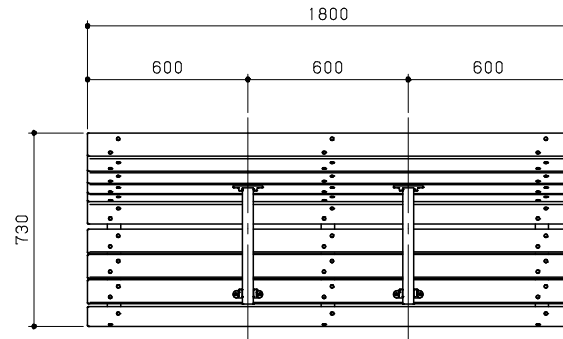
平面図 S = 1 / 20
