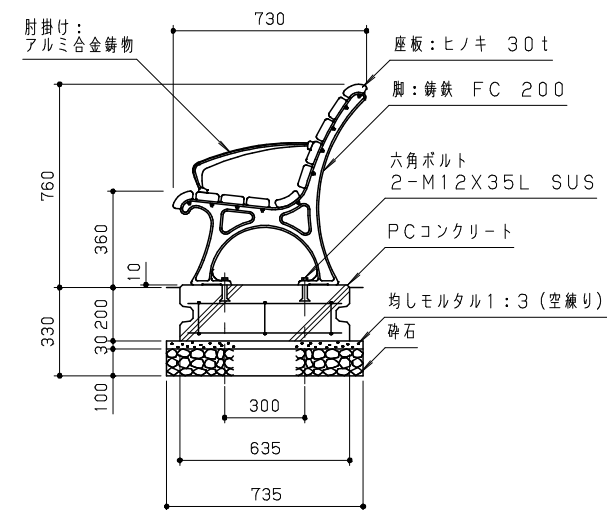
側面図 S = 1 / 20
