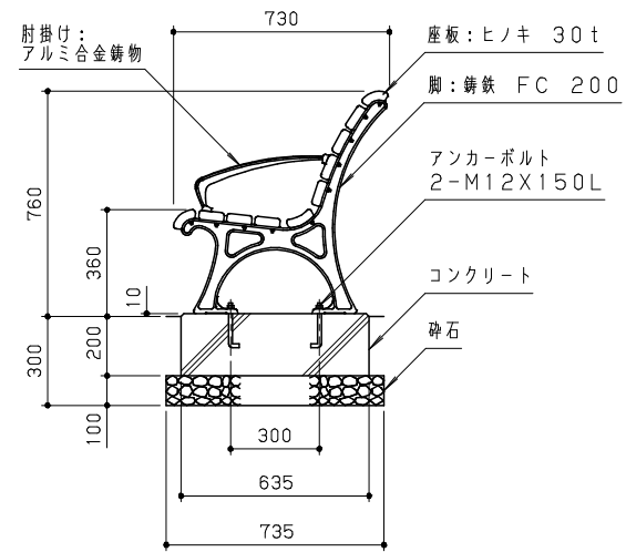
側面図 S = 1 / 20
