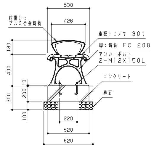
側面図 S = 1 / 20
