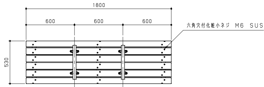
平面図 S = 1 / 20
