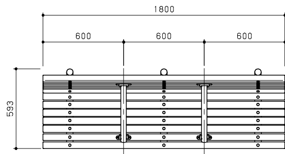
平面図 S = 1/20
