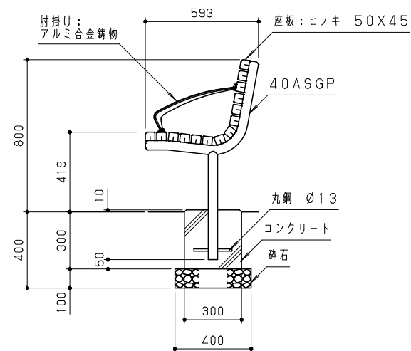
側面図 S = 1/20
