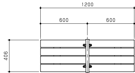
平面図 S = 1 / 20
