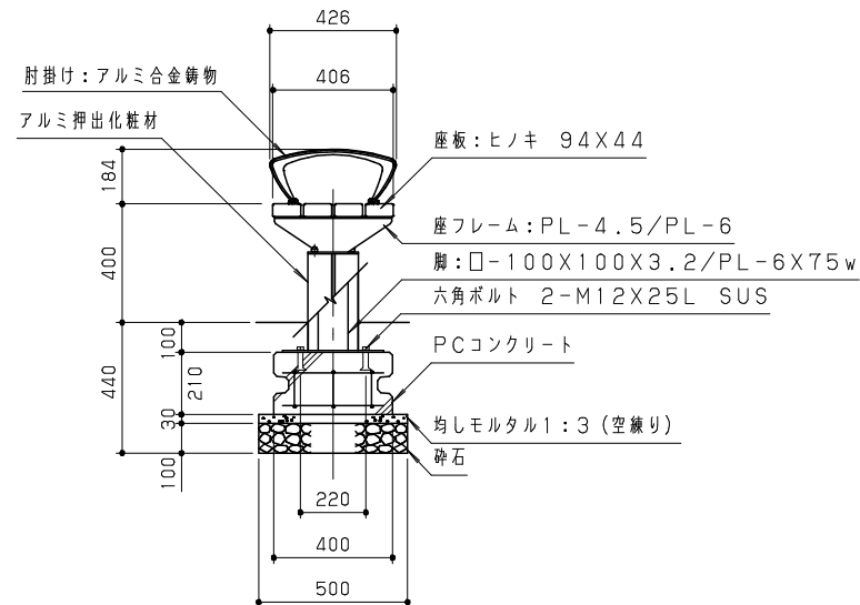
側面図 S = 1 / 20
