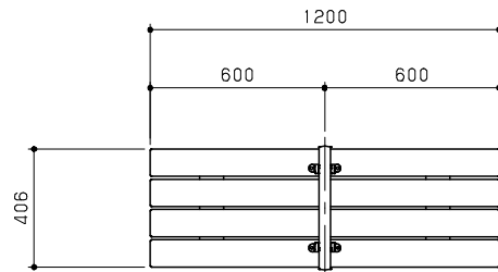
平面図 S = 1 / 20
