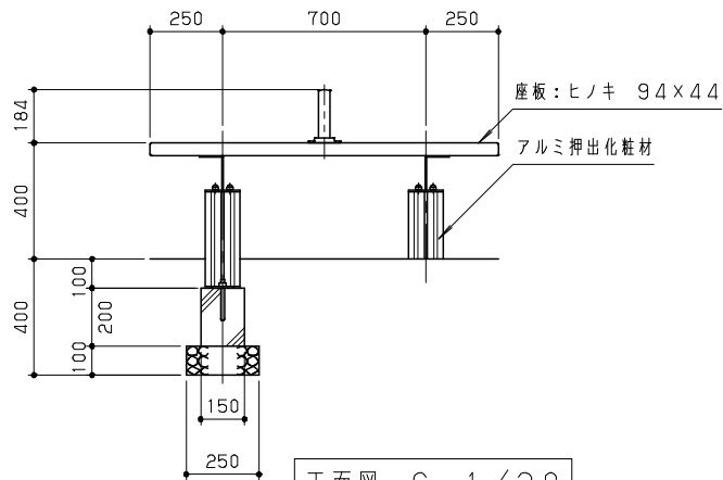
正面図 S = 1 / 20
