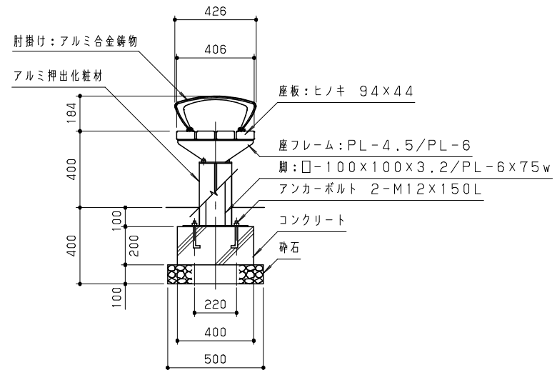
側面図 S = 1 / 20
