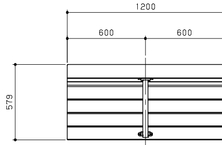
平面図 S = 1 / 20
