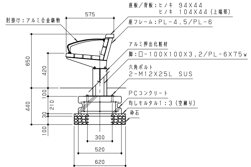
側面図 S = 1 / 20
