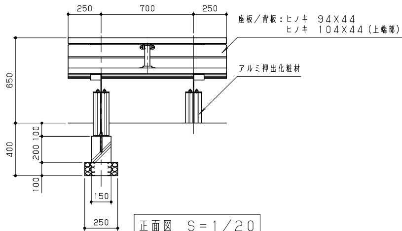
正面図 S = 1 / 20
