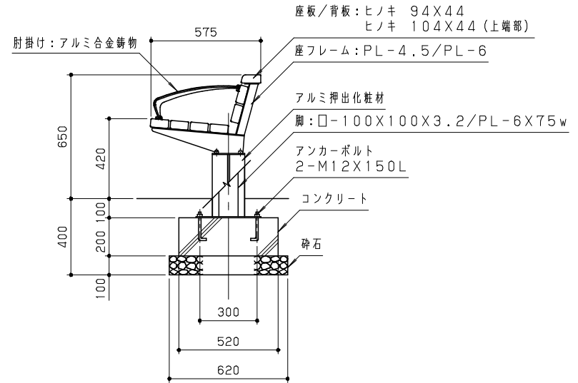
側面図 S = 1 / 20
