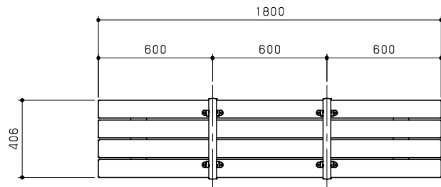
平面図 S=1/20
