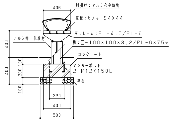
側面図 S=1/20
