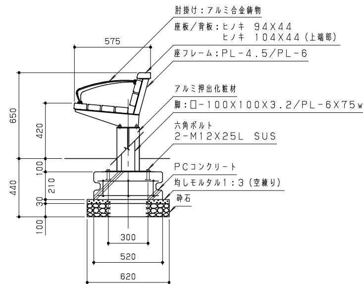
側面図 S = 1 / 20
