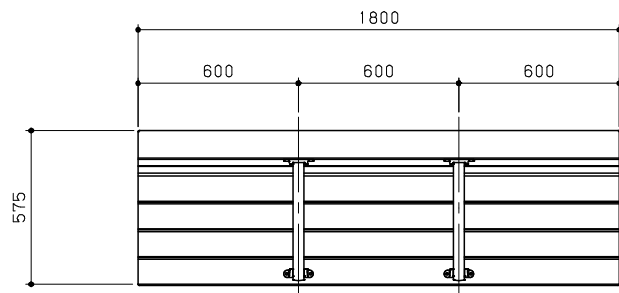
平面図 S = 1 / 20
