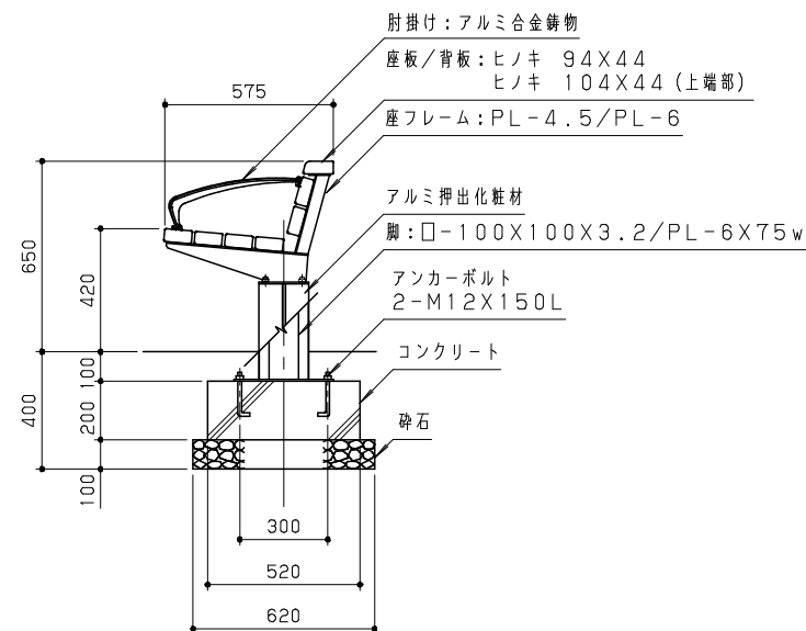
側面図 S = 1 / 20
