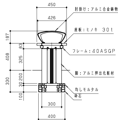
断面図 S = 1 / 20
