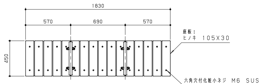
平面図 S = 1 / 20
