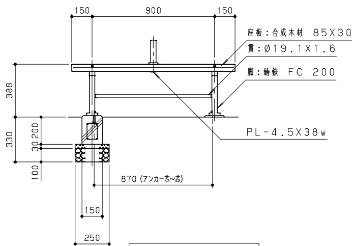
正面図 S=1/20
