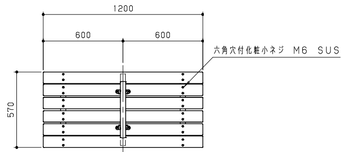
平面図 S=1/20
