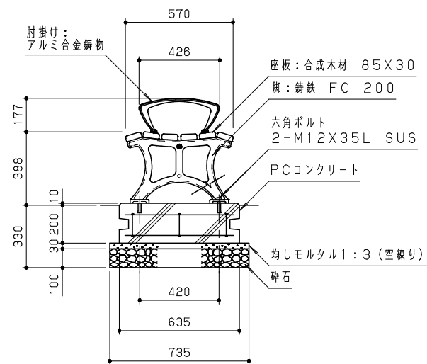
側面図 S=1/20
