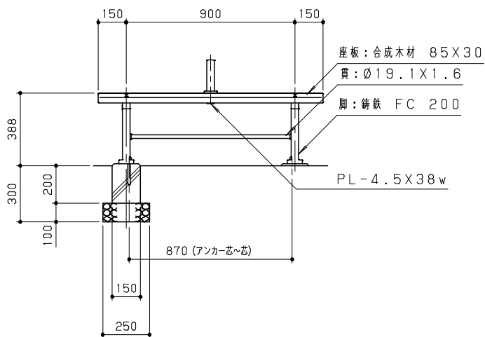
正面図 S = 1 / 20
