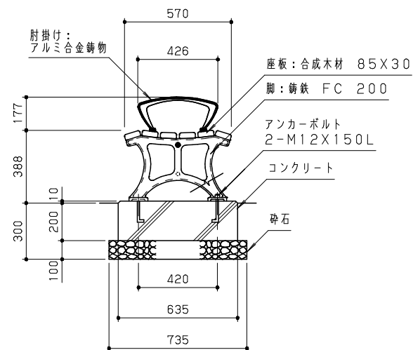
側面図 S = 1 / 20
