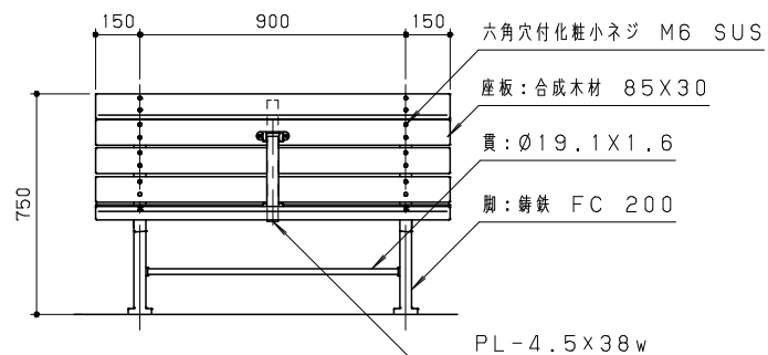
正面図 S = 1 / 20
