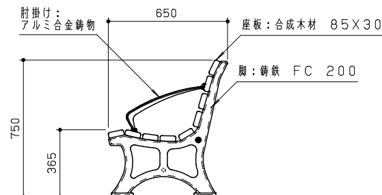
側面図 S = 1 / 20
