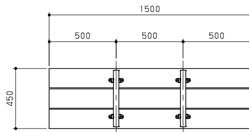
平面図 S = 1 / 20
