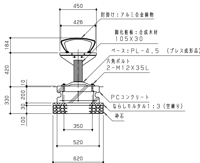
側面図 S = 1 / 20
