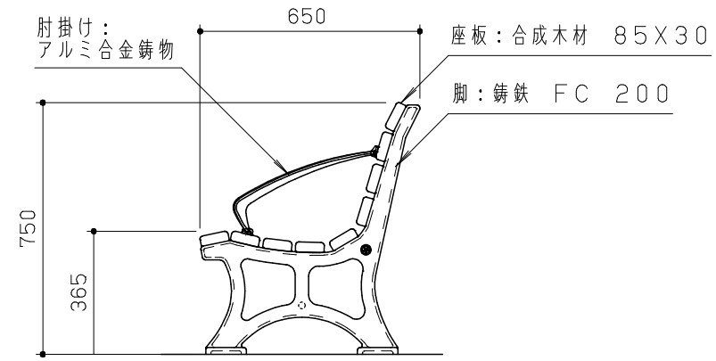
側面図 S = 1 / 20
