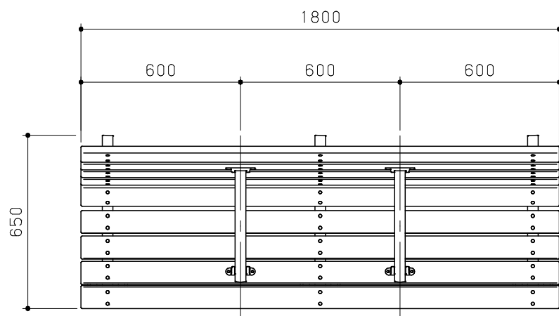
平面図 S = 1 / 20
