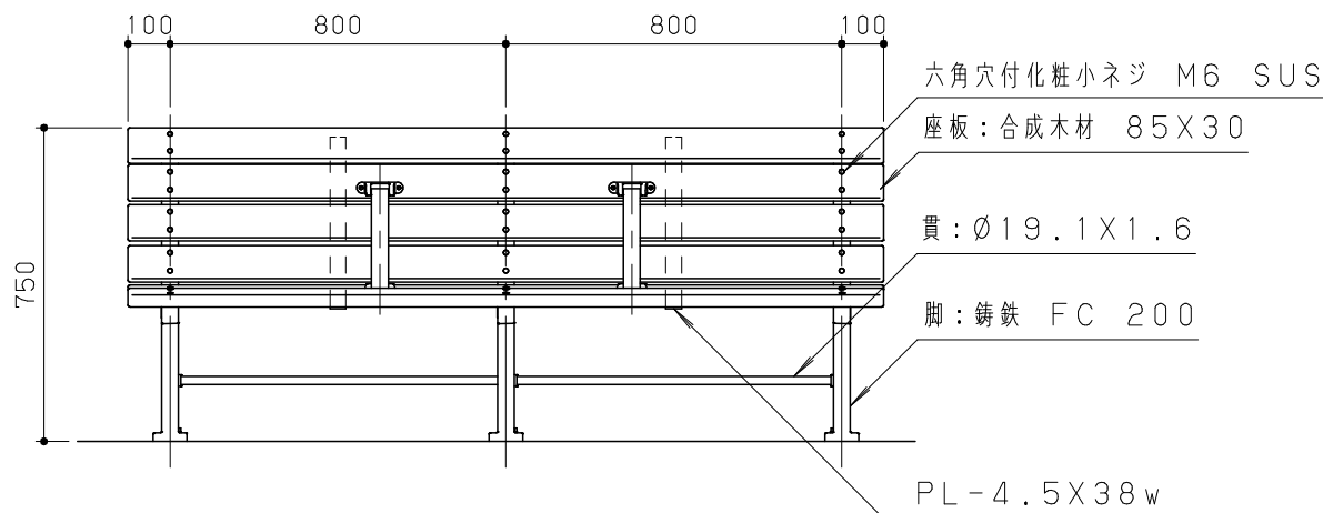
正面図 S = 1 / 20
