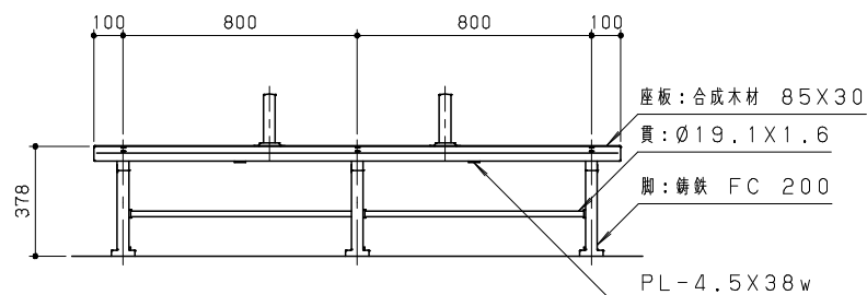
正面図 S=1/20
