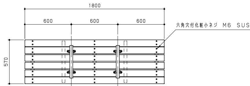
平面図 S=1/20
