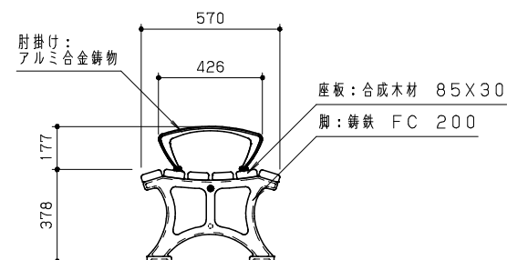
側面図 S=1/20
